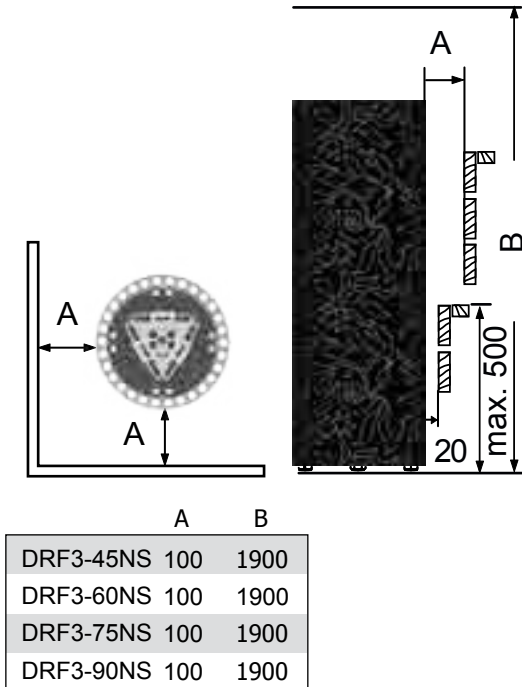
Kuva 2 | Minimisuojaetäisyydet (mm) Fig. 2 | Minimum safety distances (mm)
