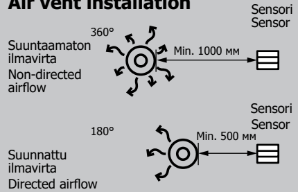
Sivunäkömä Side view
